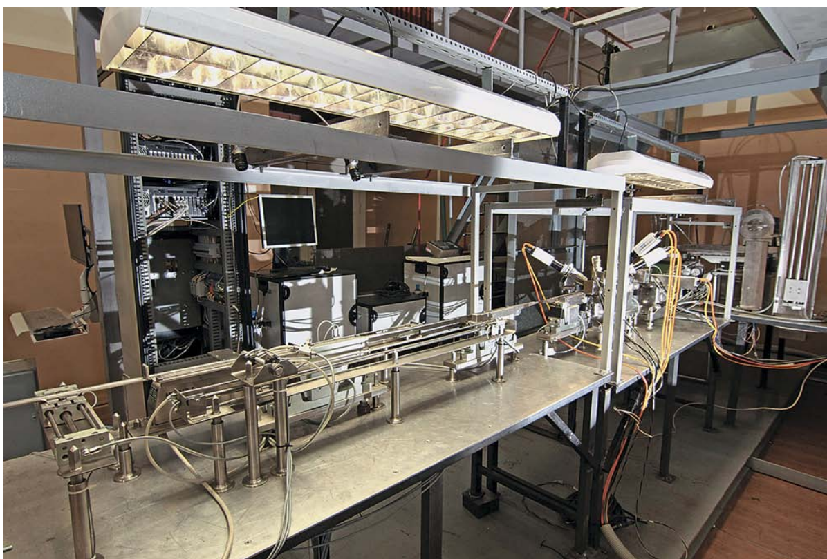
Рисунок 2.3.3 - Установка контроля качества таблеток МОКС-топлива
