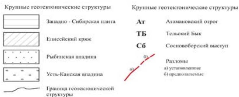
Рисунок 4.3.5.2 - Тектоническая схема района размещения
